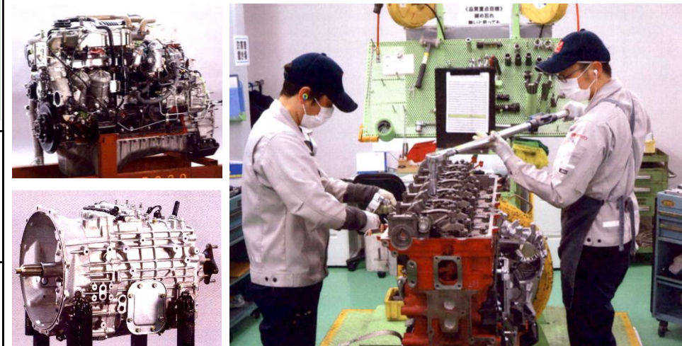
日野トラックのエンジン・トランスミッション・その他部品の再生整備
