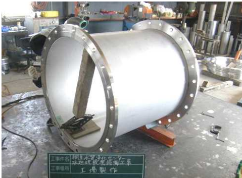
SUS900A配管製作
